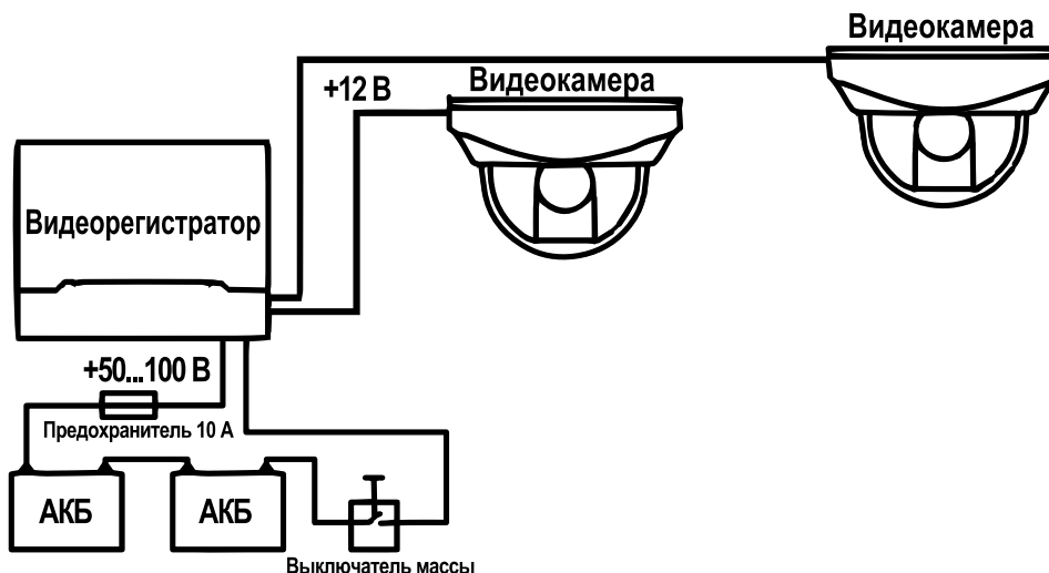
Рис. 2.2. Схема подключения
