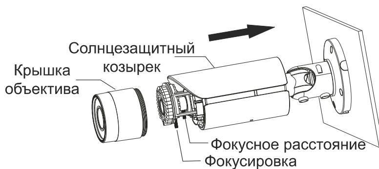
Рис. 5.4. Регулировка фокусного расстояния и фокусировки
