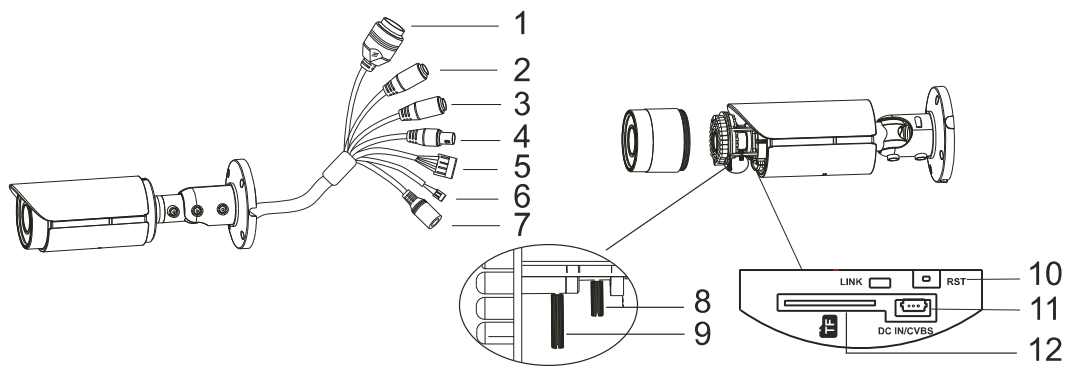
Рис. 3.1. Внешний вид
