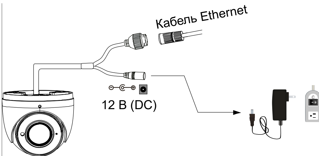
Рис. 3.2. Подключение кабелей
