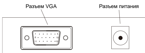
Рис. 1.1. Разъемы монитора
