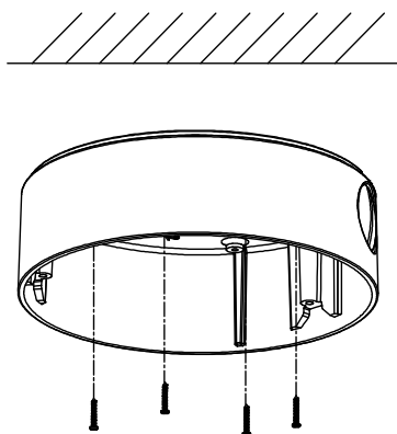
Рис. 2.2. Крепление корпуса к потолку
