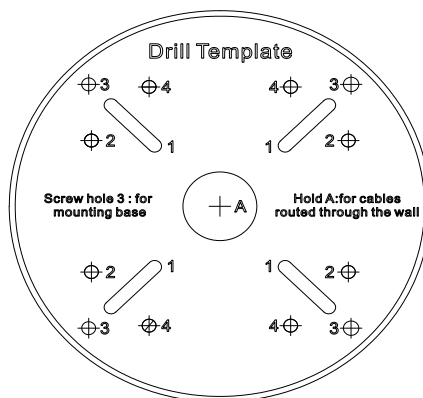
Рис. 2.1. Монтажный шаблон
