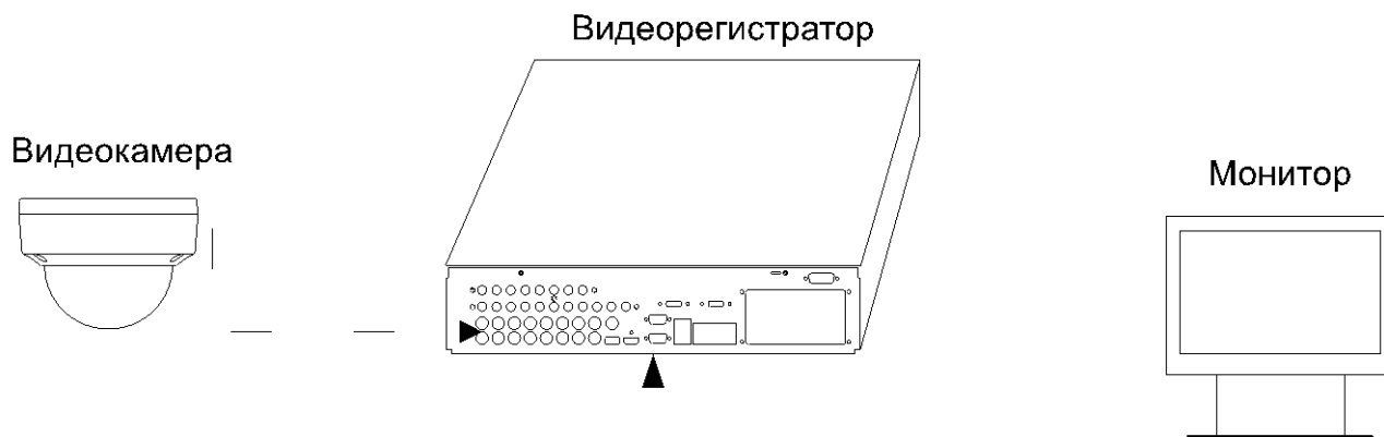
Рис. 3.1. Схема подключения
