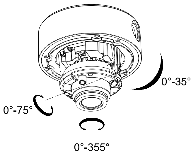
Рис. 2.4. Настройка поля зрения
