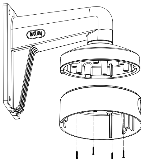
Рис. 2.6. Крепление корпуса видеокамеры к настенному кронштейну
