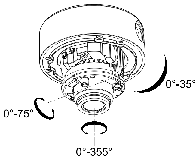
Рис. 2.7. Настройка поля зрения
