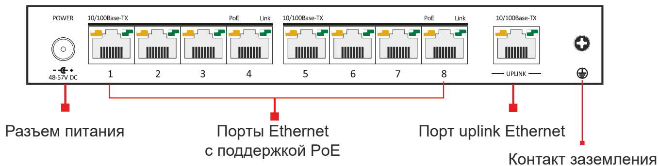
Рис. 2.3. Задняя панель
