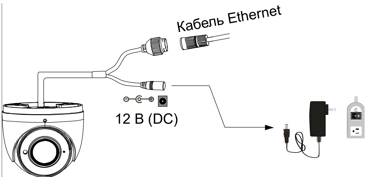
Рис. 3.2. Подключение кабелей
