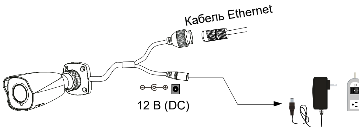
Рис. 3.2. Подключение кабелей
