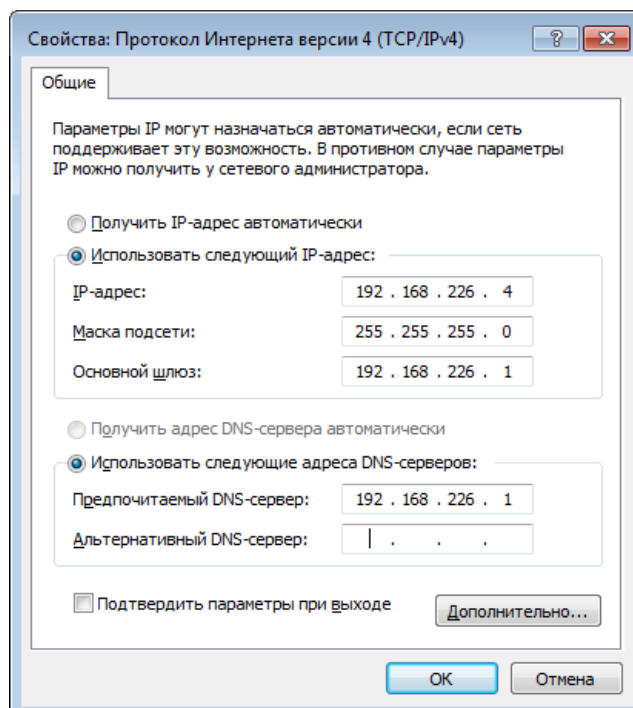
Рис. 6.6. Настройки IP-протокола
