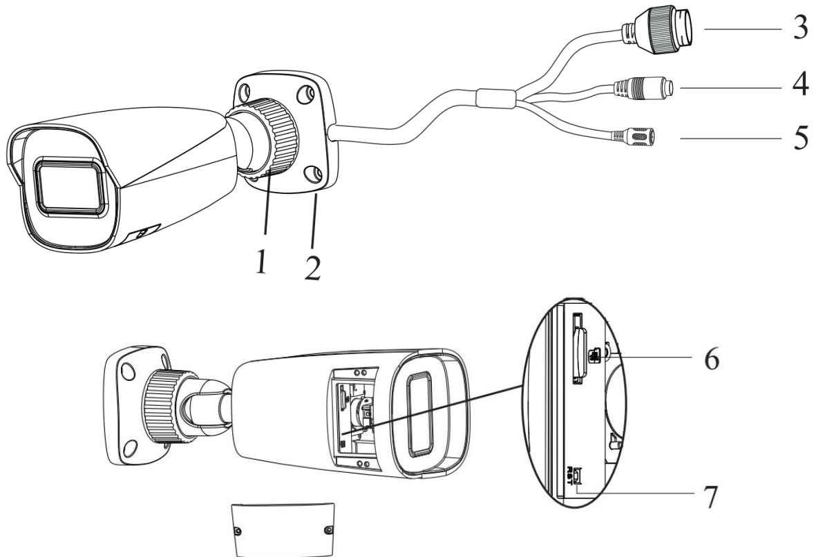
Рис. 3.1 Внешний вид
