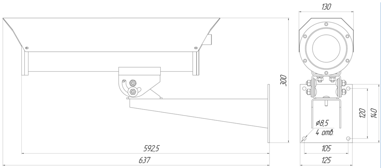
Рис. 3.2. Размеры термостат с крепежно-юстировочным устройством
