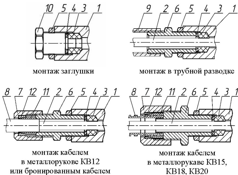
Рис. 4.4. Различные вводные устройства
