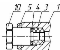
монтаж заглушки
