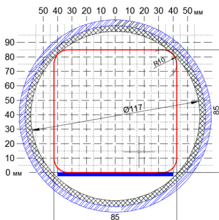
Рисунок 4.4 – Сечение термокожуха
