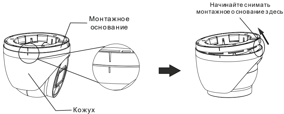
Рис. 5.1. Снятие монтажного основания
