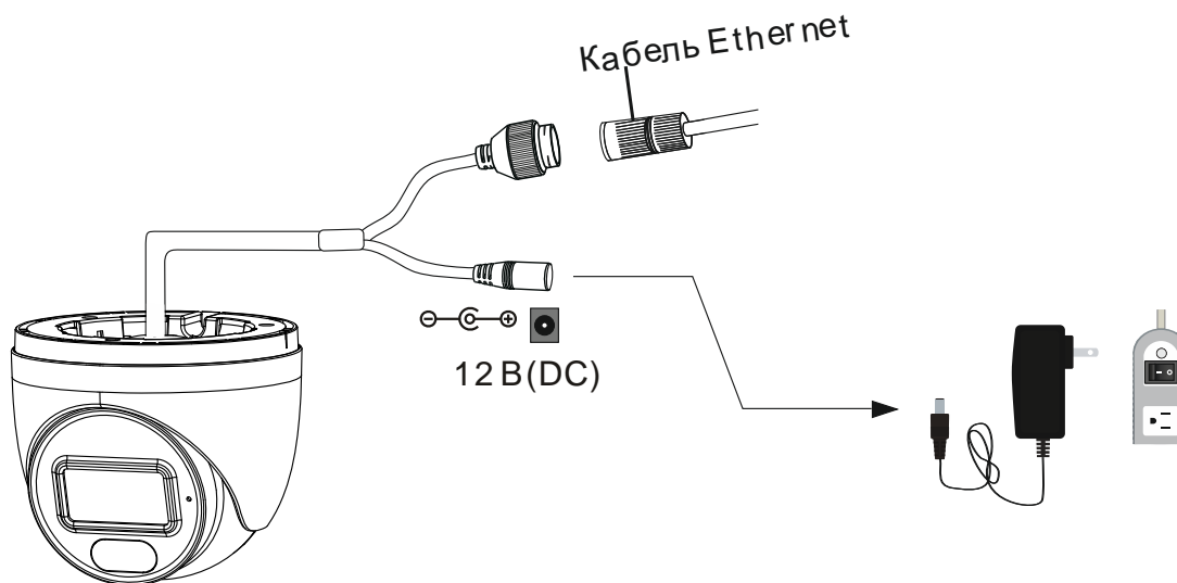
Рис. 3.2. Подключение кабелей
