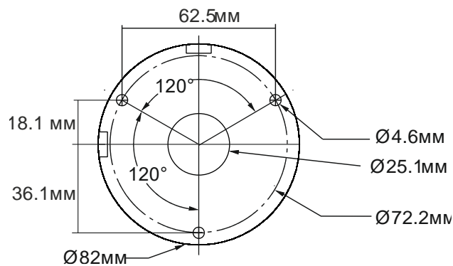
Рис. 5.2. Размеры монтажного шаблона
