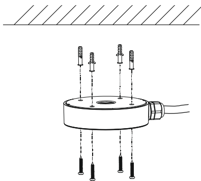
Рис. 5.7. Крепление монтажной коробки
