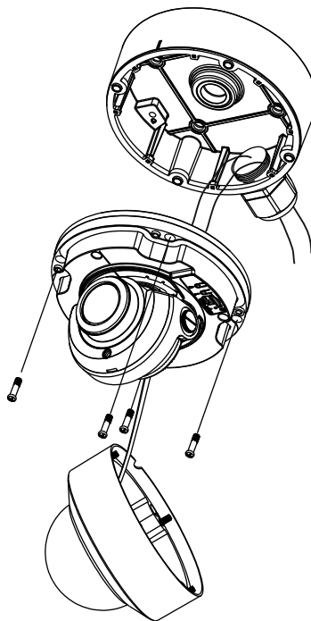
Рис. 5.8. Крепление видеокамеры к монтажной коробке
