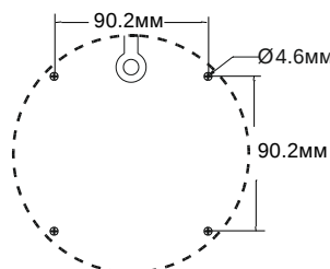
Рис. 5.1. Монтажный шаблон
