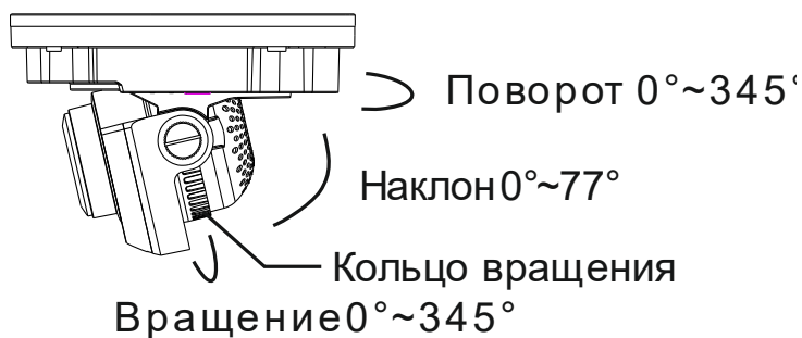
Рис. 5.5. Регулировка направления обзора
