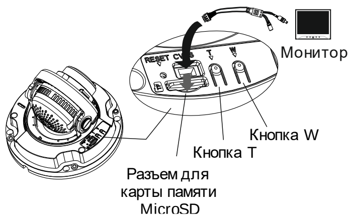
Рис. 5.4. Установка карты памяти microSD и регулировка фокусного расстояния
