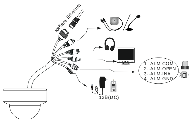
Рис. 3.2. Подключение кабелей
