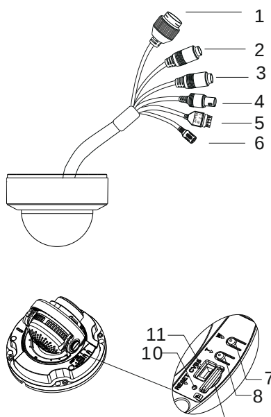
Рис. 3.1. Внешний вид
