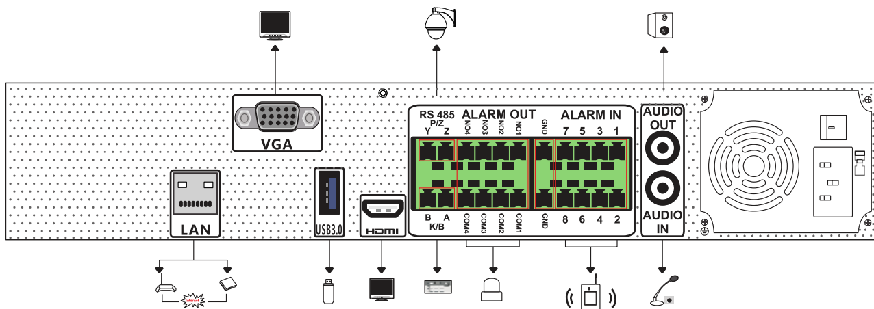
Рис. 1.1. Задняя панель LTV RNE-161 01
