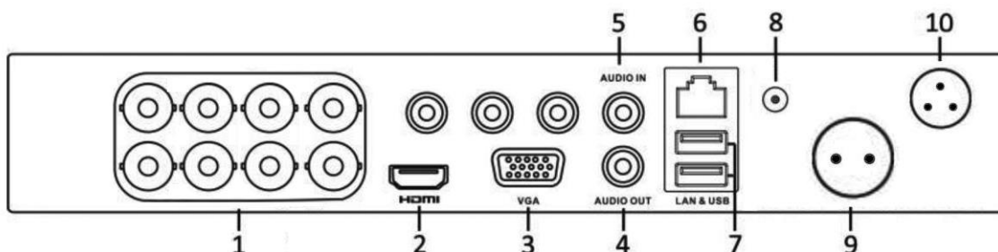
Рис. 2.1. Разъемы на задней панели видеорегистратора
