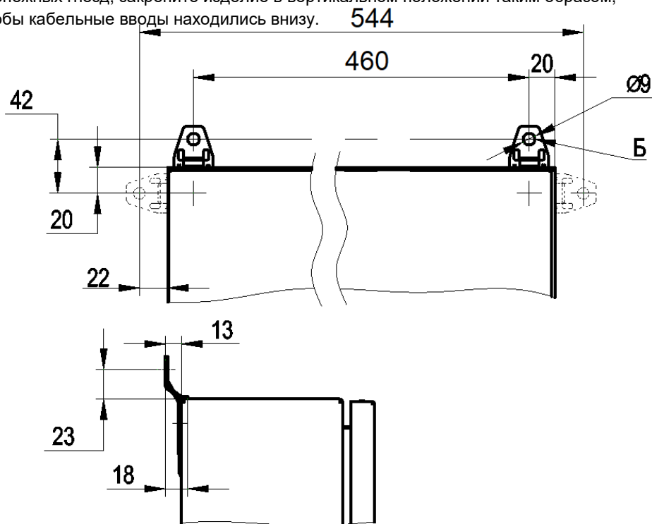
Рисунок 4 – пример установки кронштейнов
