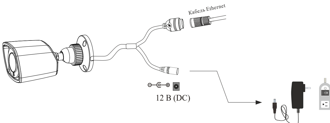
Рис. 3.2. Подключение кабелей
