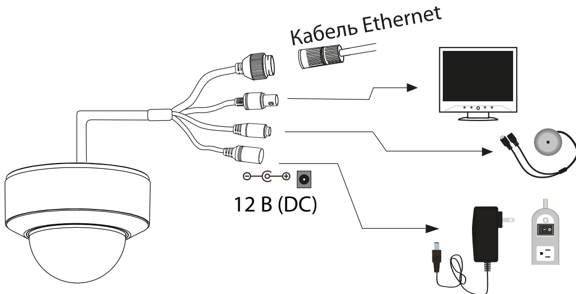
Рис. 3.2. Подключение кабелей
