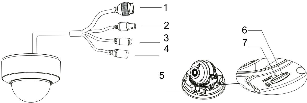
Рис. 3.1. Внешний вид
