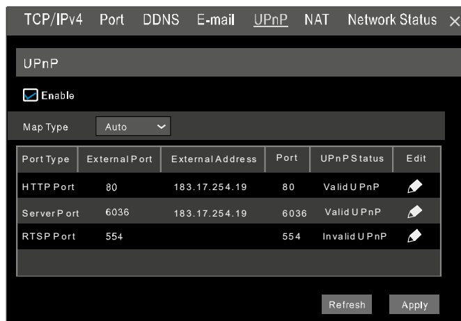
Рис. 1.9. Меню настроек UPnP
