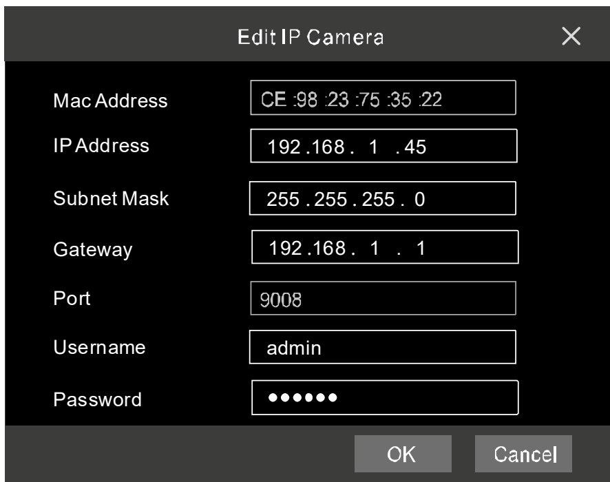
Рис. 1.6. Меню редактирования сетевых настроек IP-видеокамеры
