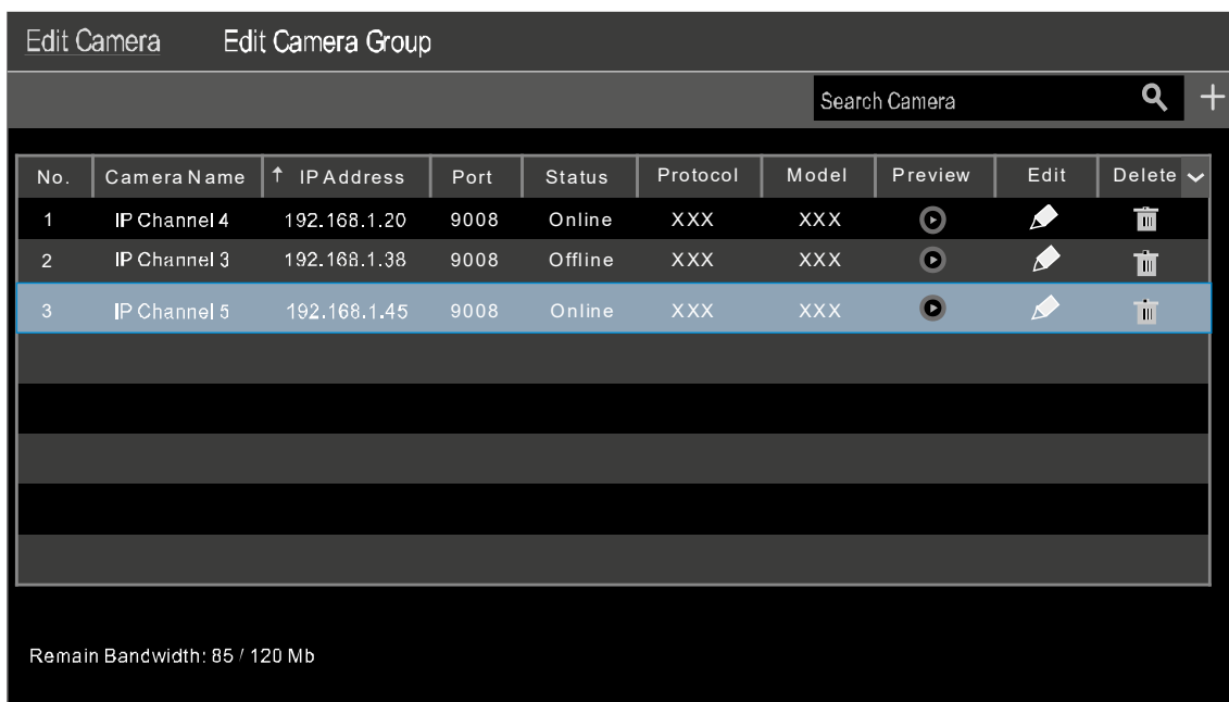
Рис. 1.7. Меню редактирования списка IP-видеокамер
