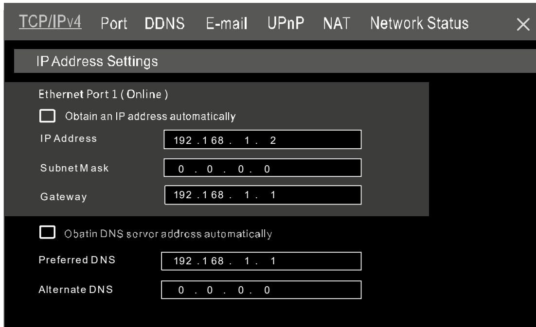
Рис. 1.4. Меню настроек TCP/IP
