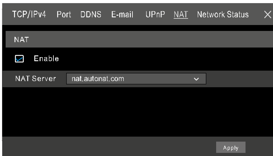
Рис. 1.10. Меню настроек NAT
