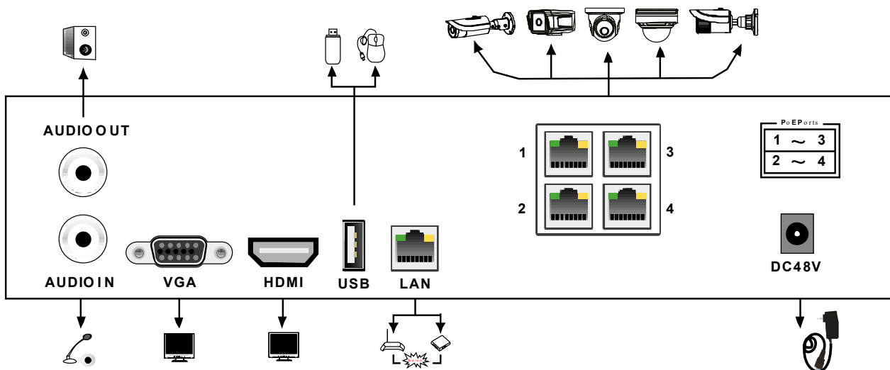
Рис. 1.1. Задняя панель IP-видеорегистратора LTV RNE-040 0G
