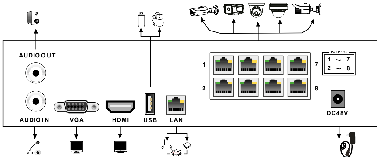
Рис. 1.2. Задняя панель IP-видеорегистратора LTV RNE-080 0G
