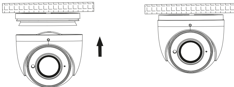
Рис. 5.4. Завершение монтажа
