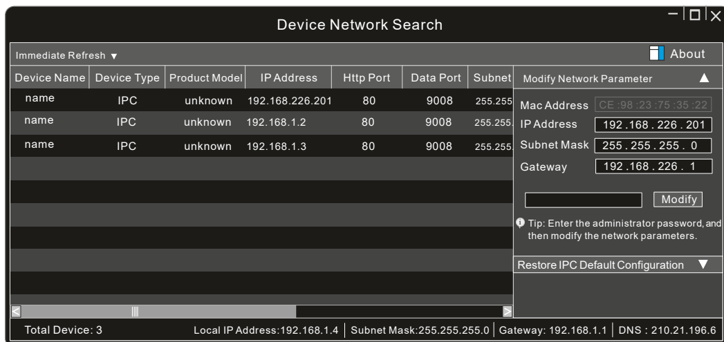
Рис. 6.2. Интерфейс IP-Tool
