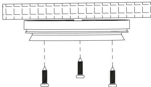
Рис. 5.3. Крепление монтажного основания
