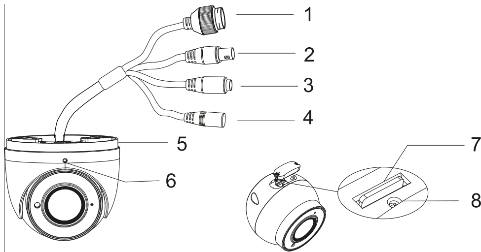
Рис. 3.1. Внешний вид
