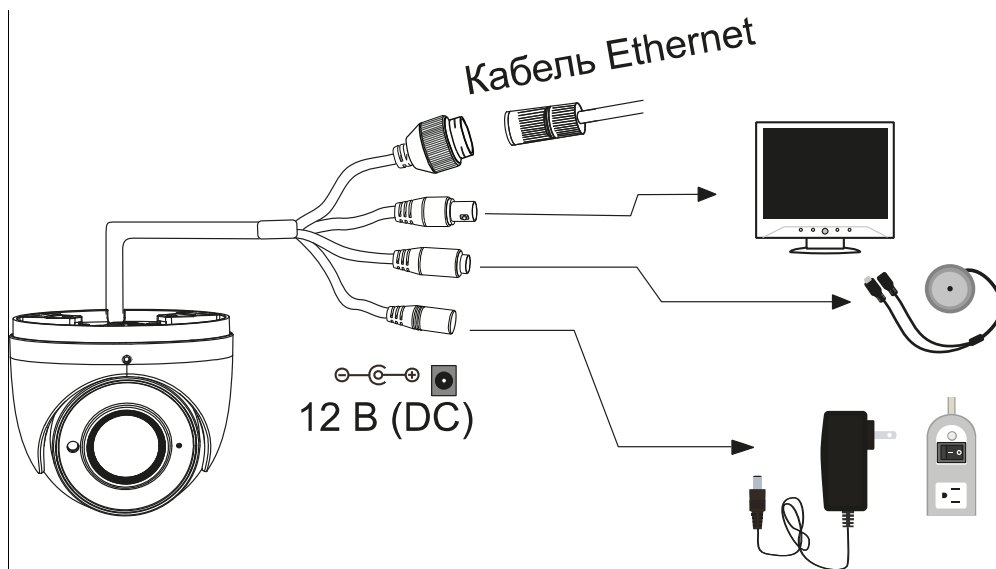
Рис. 3.2. Подключение кабелей
