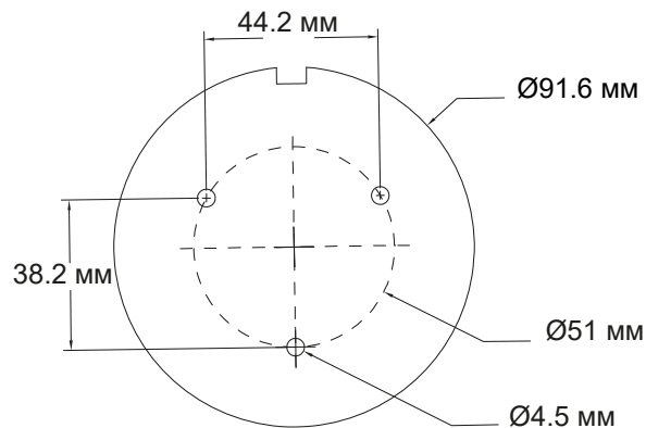
Рис. 5.2. Размеры монтажного шаблона
